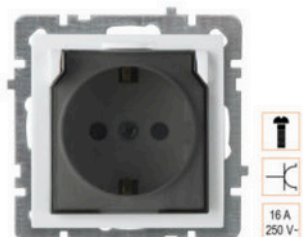
24 XX 04 20 Utičnica Sa Poklopcem, Uzemljenjem I Zaštitom Za Djecu Child Protected Earthed Socket with Cover Розетка с Крышкой, Зазем и 3Ш
