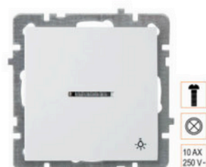
24 XX 04 06 Prekidač Za Svjetlo Sa Osvjetljenjem Illuminated Light Switch Выкл. Кнопка с Подсвет
