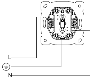
Bağlantı Şeması
