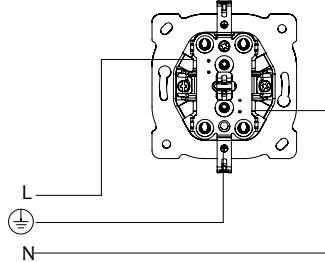
Bağlantı Şeması
