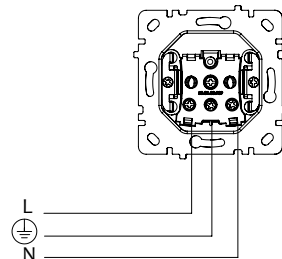
Bağlantı Şeması
